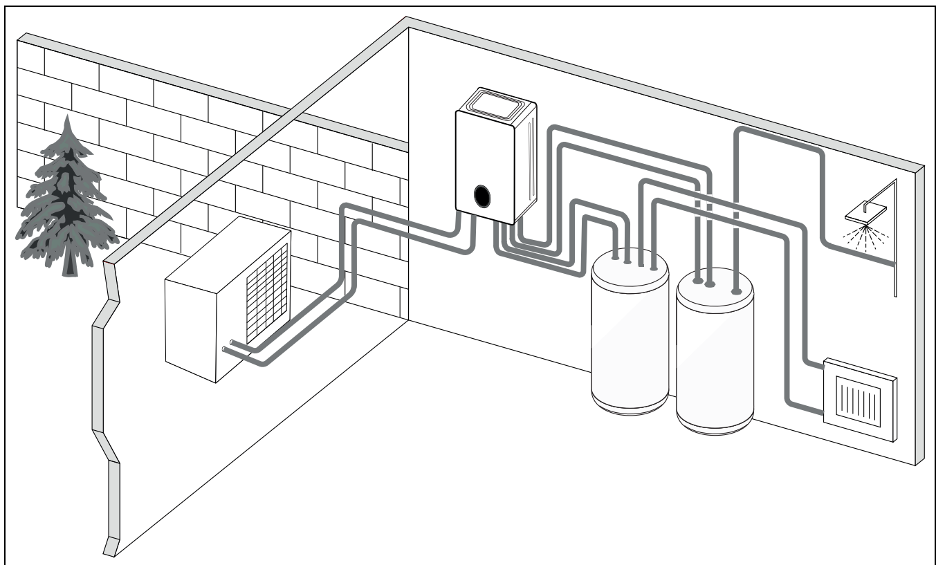
Sl.7 Toplotna črpalka AW OR, notranja enota Compress 5800i 12 E s potopljenim grelnikom in zunanjim boilerjem
