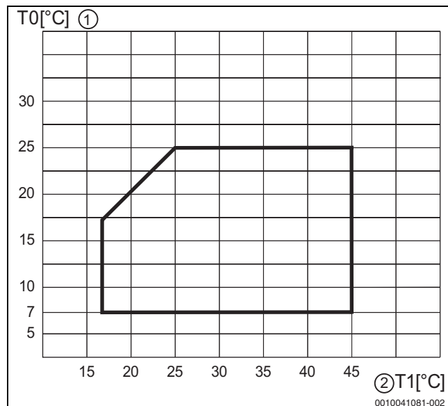
Sl.5 Toplotna črpalka v načinu hlajenja
