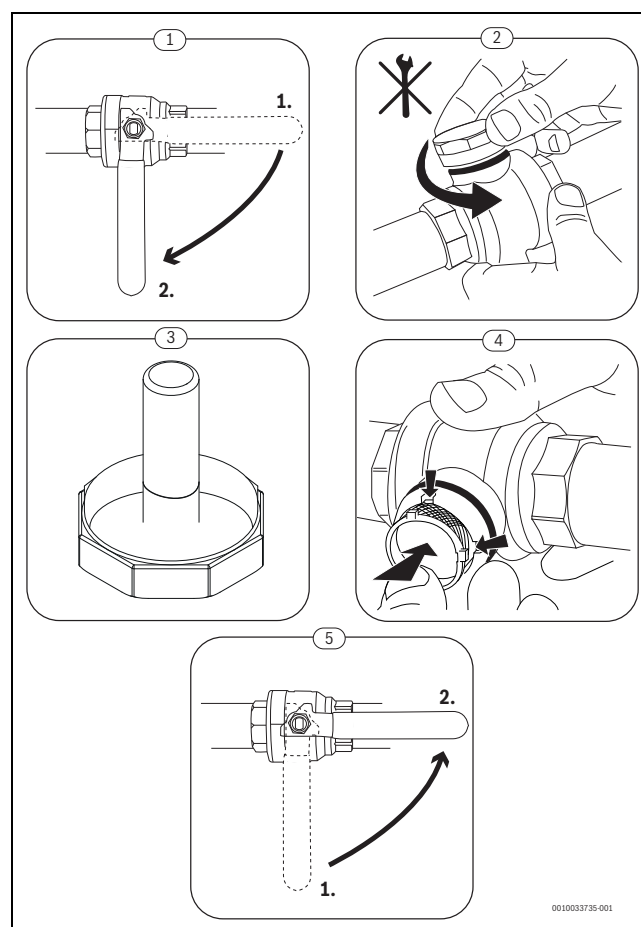
Sl.14 Čiščenje filtra
