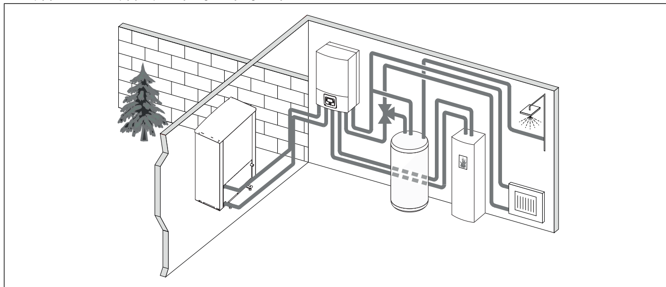
Sl.3 Toplotna črpalka Compress 6000 AW, notranja enota AWB brez dodatnega električnega grelnika, zunanji bojler in dodatni zunanji grelnik
